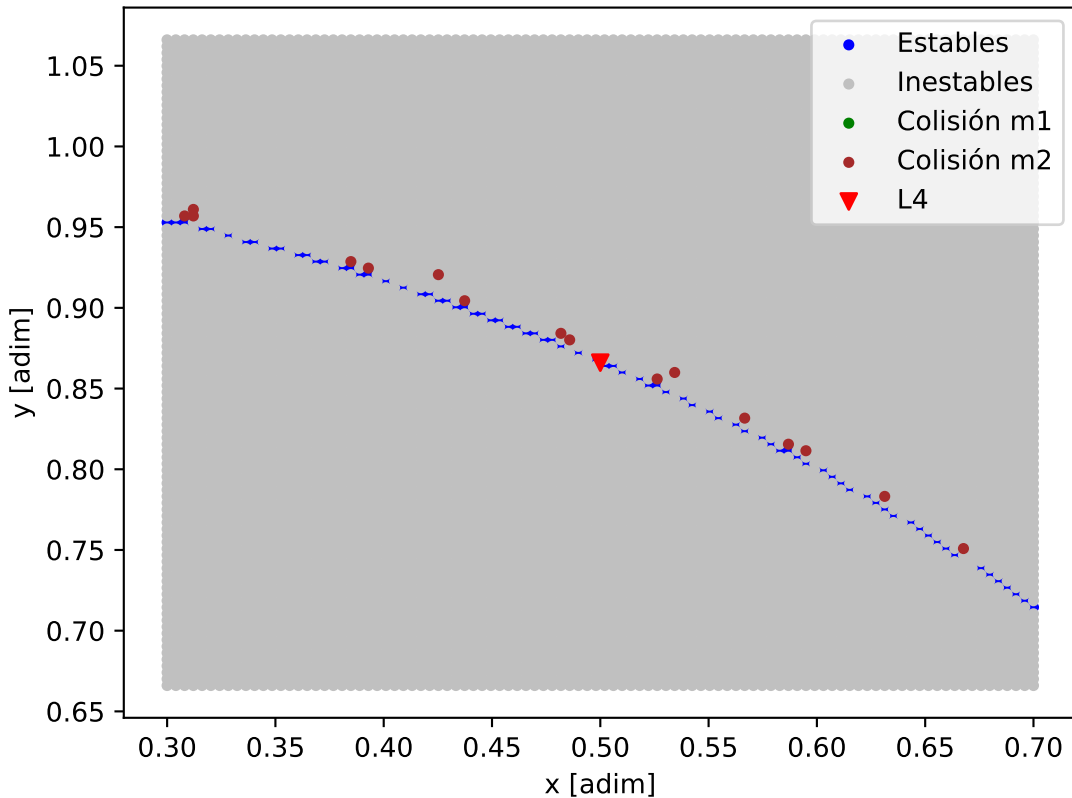
Mapa de estabilidad - Barnard's_star_Barnard_c
