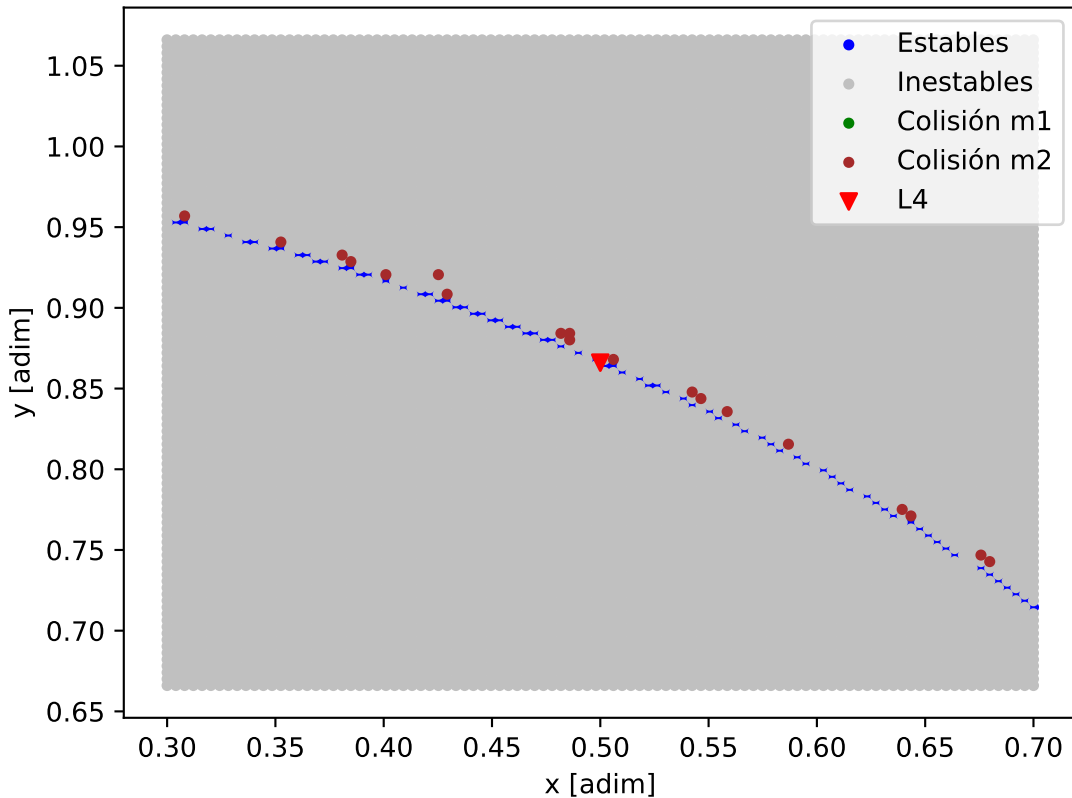
Mapa de estabilidad - Barnard's_star_Barnard_d
