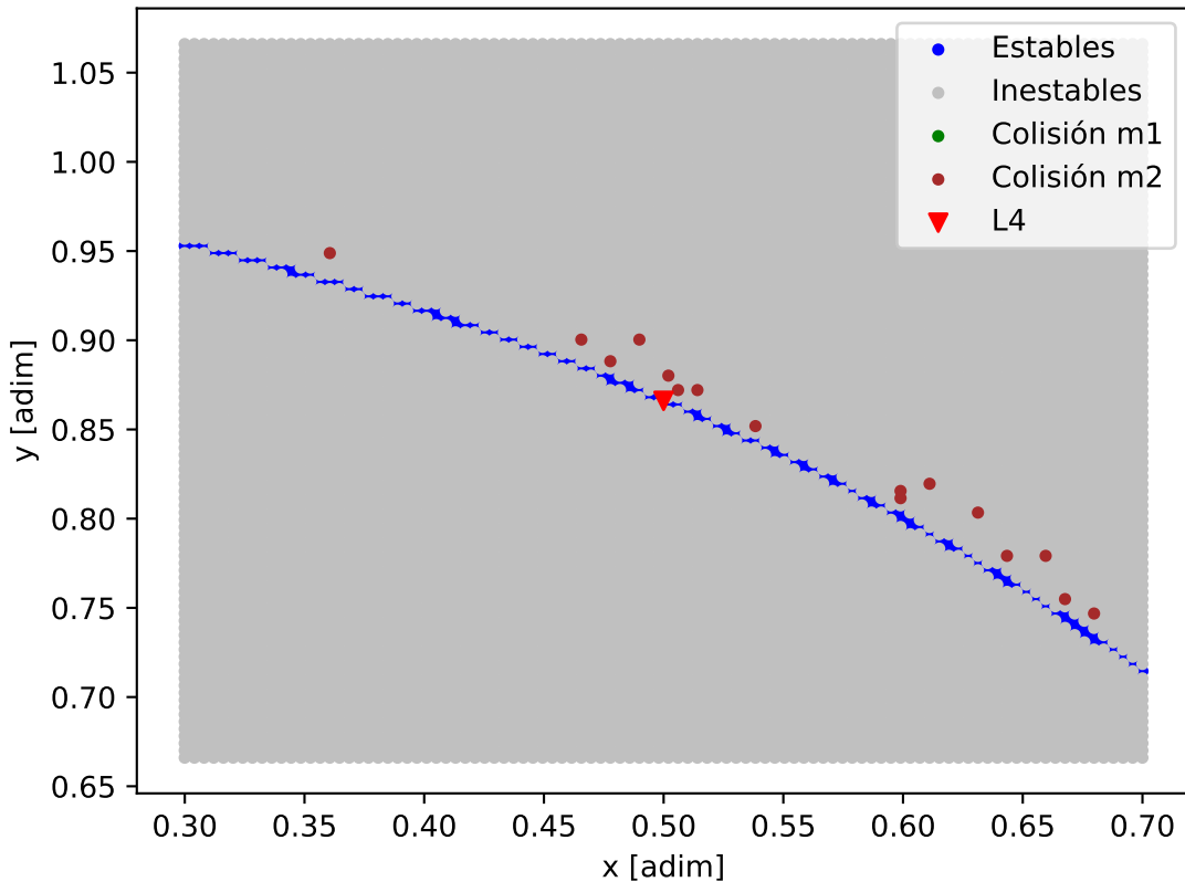
Mapa de estabilidad - GJ_1061_GJ_1061_b
