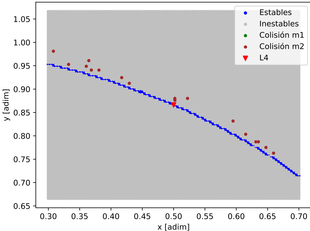
Mapa de estabilidad - GJ_1061_GJ_1061_c
