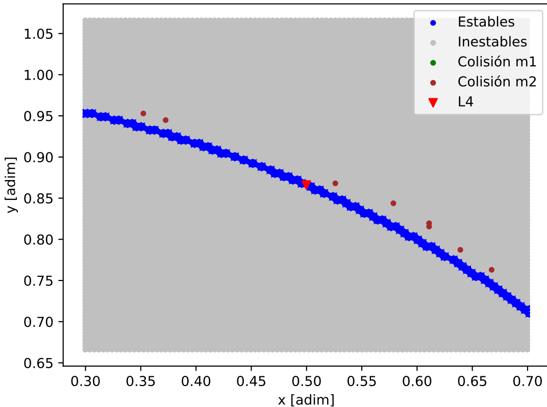
Mapa de estabilidad - GJ_163_GJ_163_d
