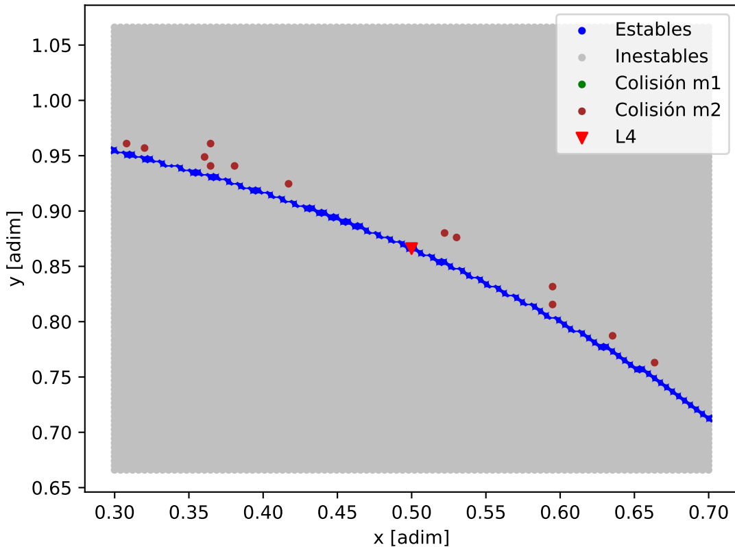
Mapa de estabilidad - GJ_180_GJ_180_d
