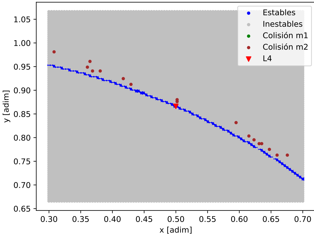
Mapa de estabilidad - GJ_3138_GJ_3138_d
