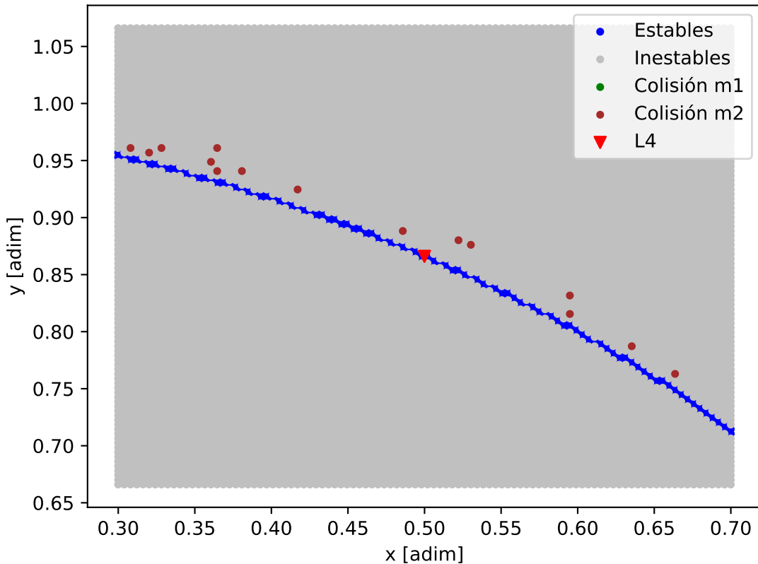
Mapa de estabilidad - GJ_3293_GJ_3293_d
