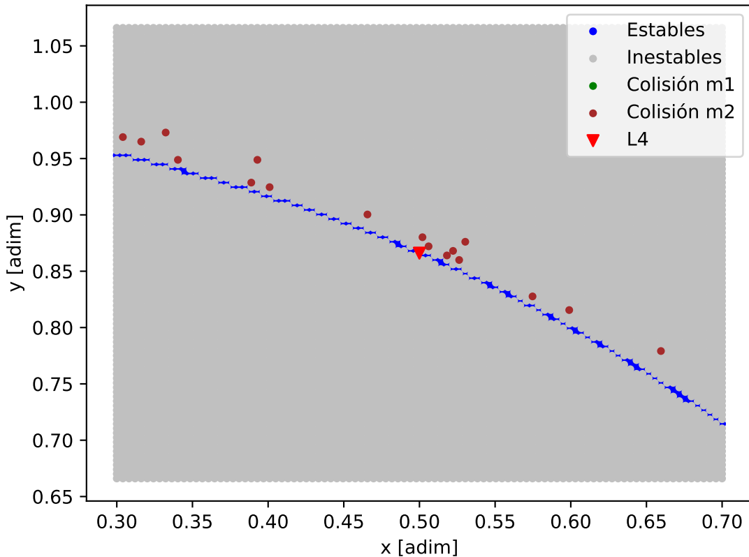
Mapa de estabilidad - GJ_3293_GJ_3293_e
