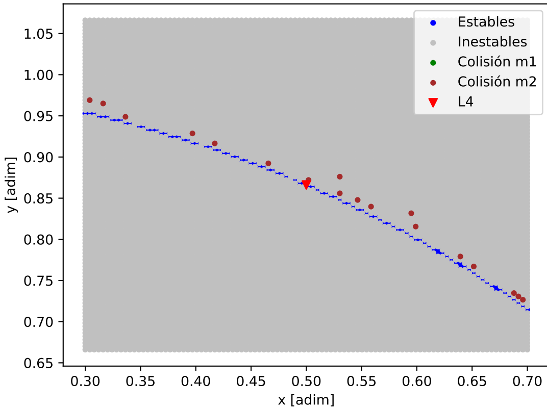
Mapa de estabilidad - GJ_357_GJ_357_b
