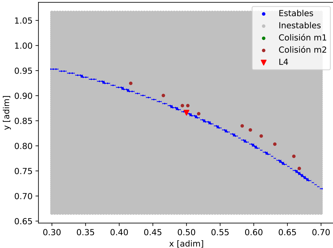
Mapa de estabilidad - GJ_357_GJ_357_c
