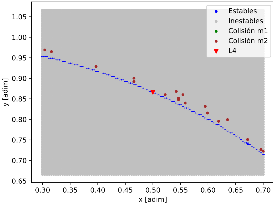
Mapa de estabilidad - GJ_3998_GJ_3998_b
