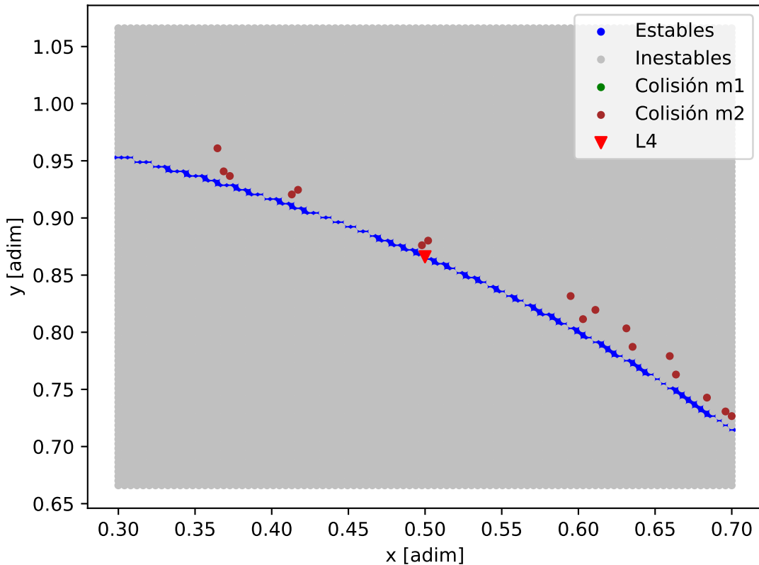
Mapa de estabilidad - GJ_3998_GJ_3998_d
