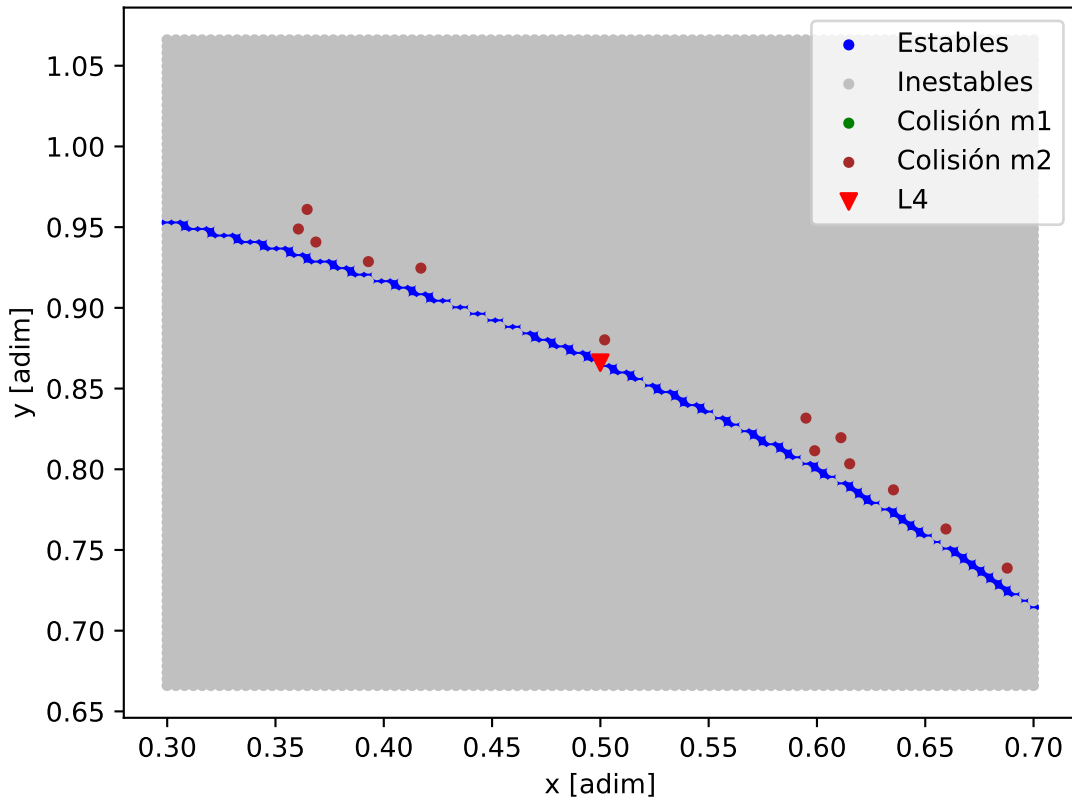
Mapa de estabilidad - GJ_433_GJ_433_b
