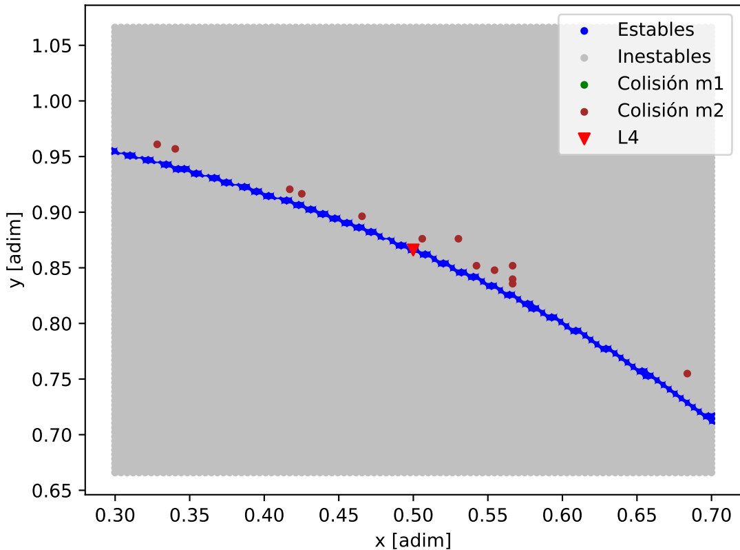
Mapa de estabilidad - GJ_581_GJ_581_c
