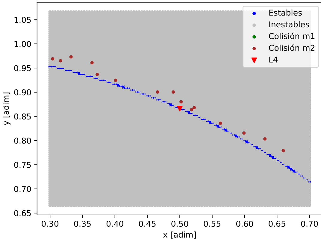
Mapa de estabilidad - GJ_581_GJ_581_e
