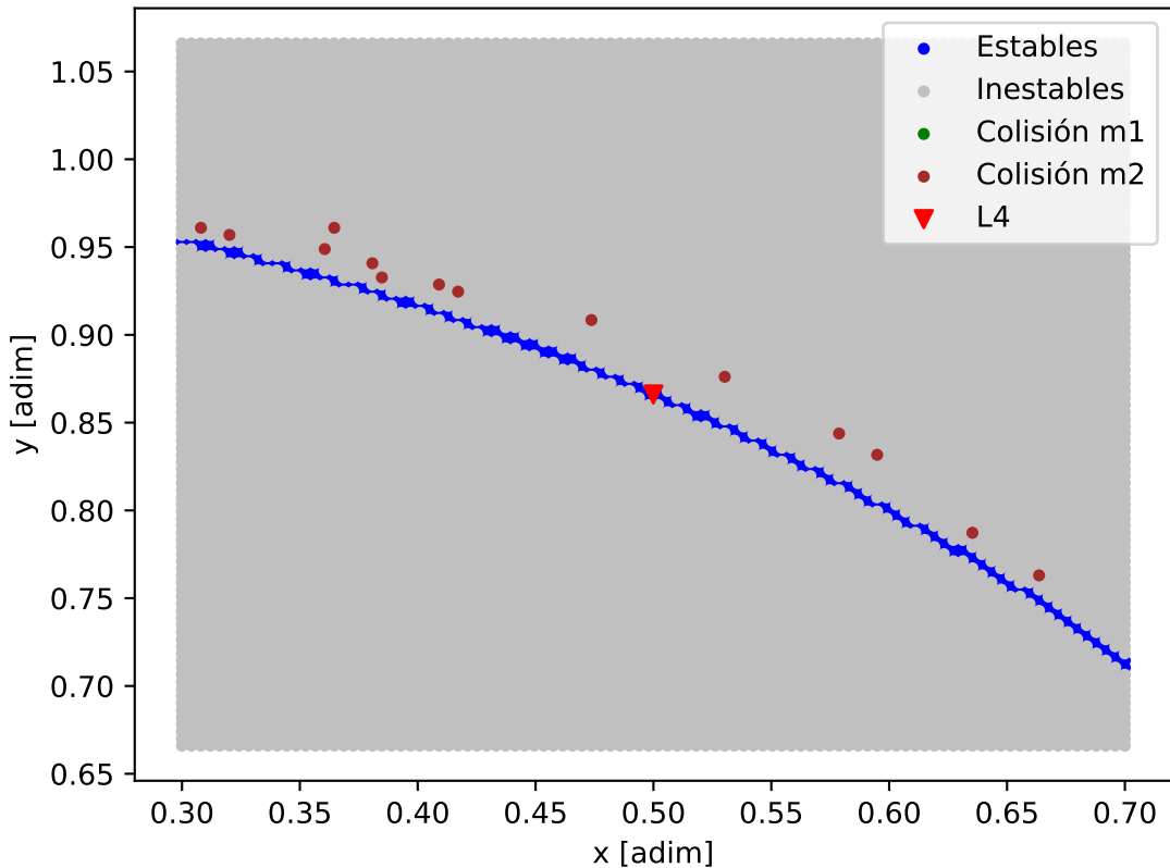
Mapa de estabilidad - GJ_667_C_GJ_667_C_b
