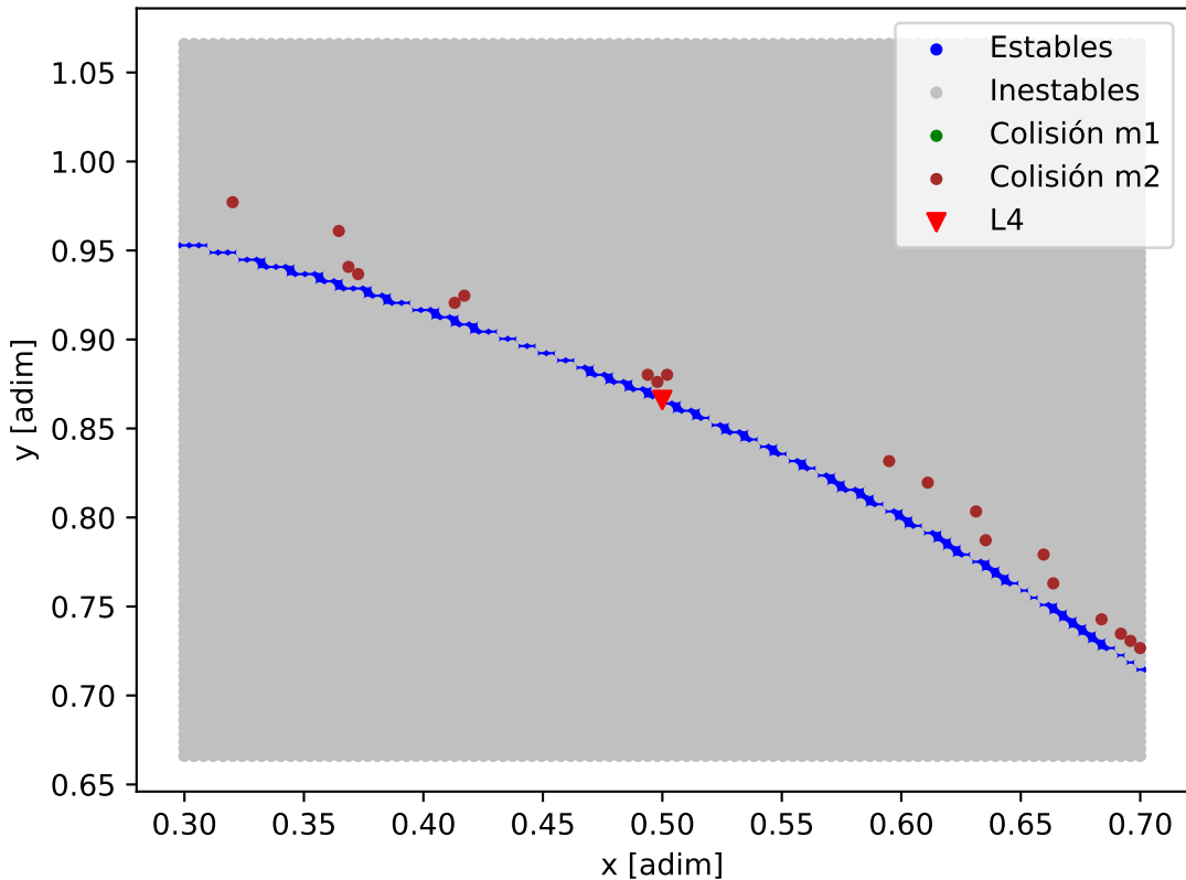
Mapa de estabilidad - GJ_667_C_GJ_667_C_c
