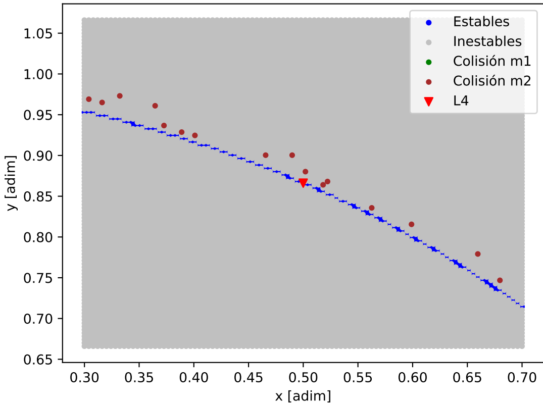
Mapa de estabilidad - GJ_667_C_GJ_667_C_f
