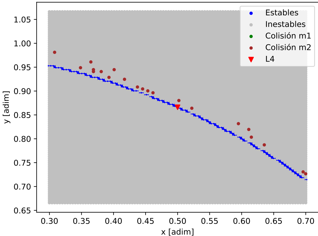
Mapa de estabilidad - GJ_667_C_GJ_667_C_g
