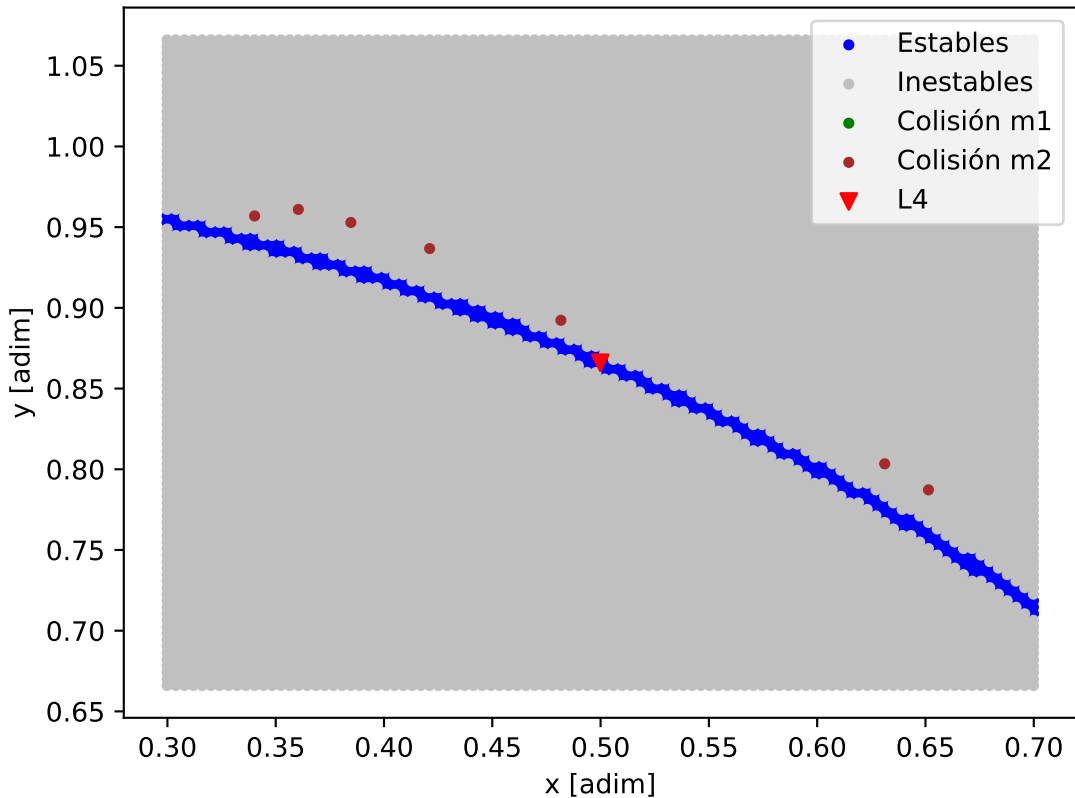
Mapa de estabilidad - GJ_876_GJ_876_e
