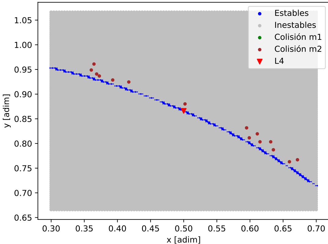
Mapa de estabilidad - GJ_887_GJ_887_d
