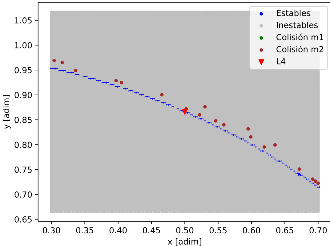
Mapa de estabilidad - K2-133_K2-133_b
