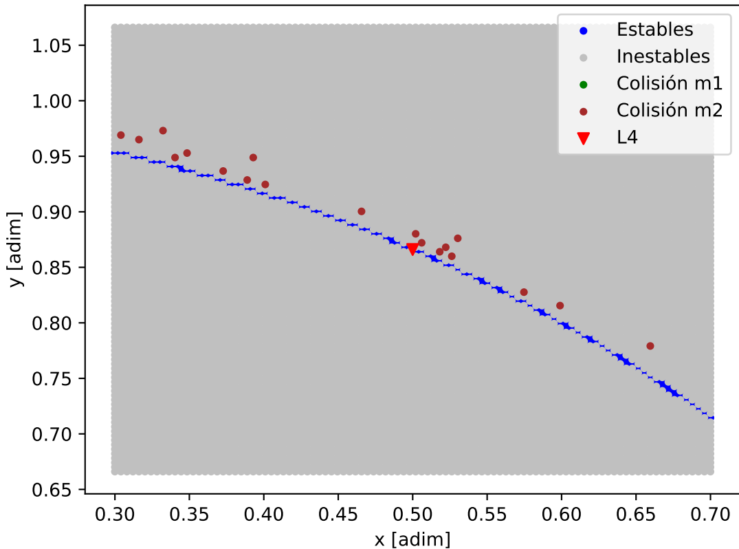
Mapa de estabilidad - K2-133_K2-133_e
