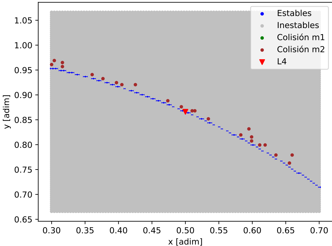
Mapa de estabilidad - K2-239_K2-239_b
