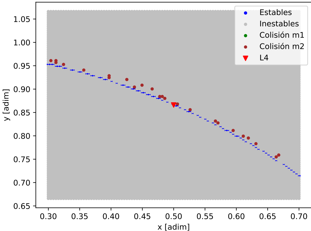
Mapa de estabilidad - K2-239_K2-239_c
