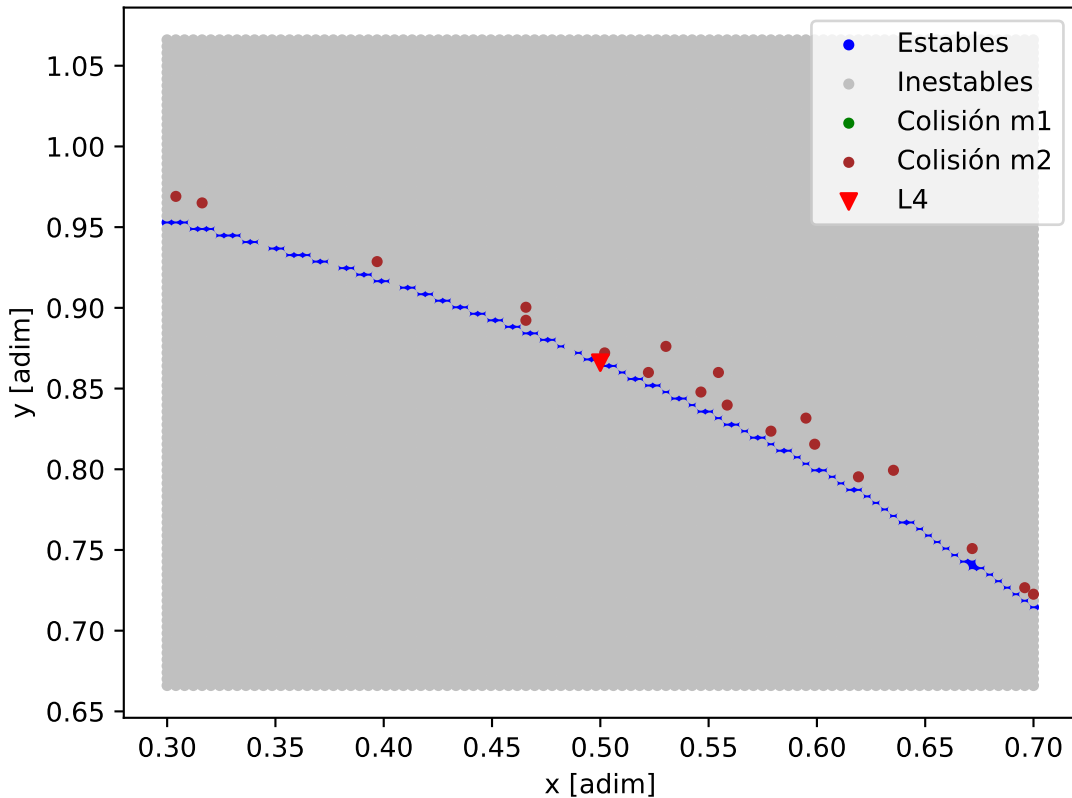
Mapa de estabilidad - K2-3_K2-3_c
