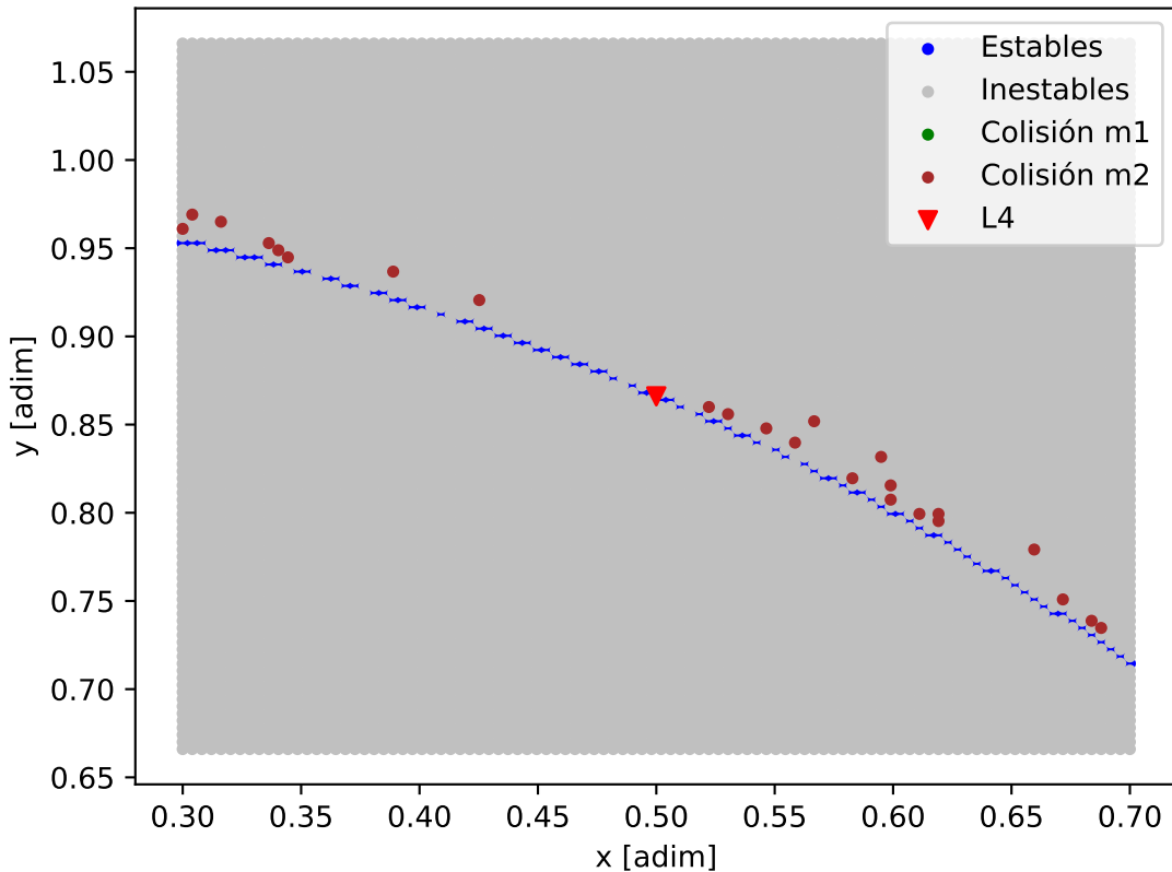
Mapa de estabilidad - K2-3_K2-3_d
