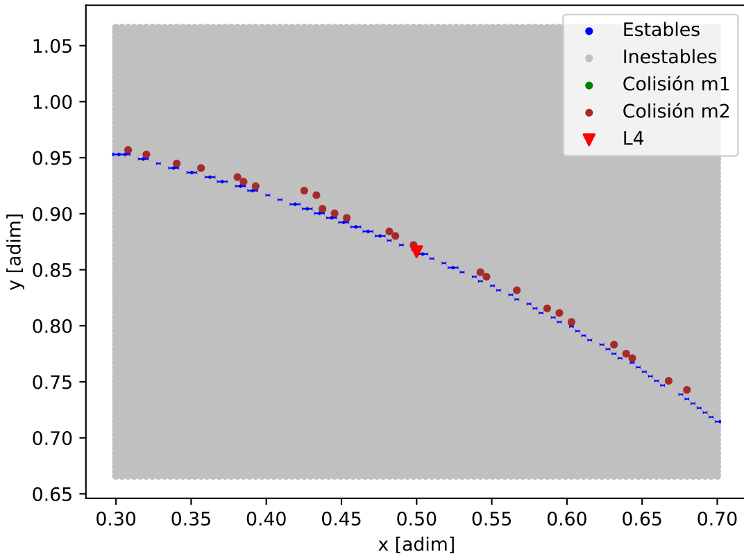
Mapa de estabilidad - Kepler-114_Kepler-114_b
