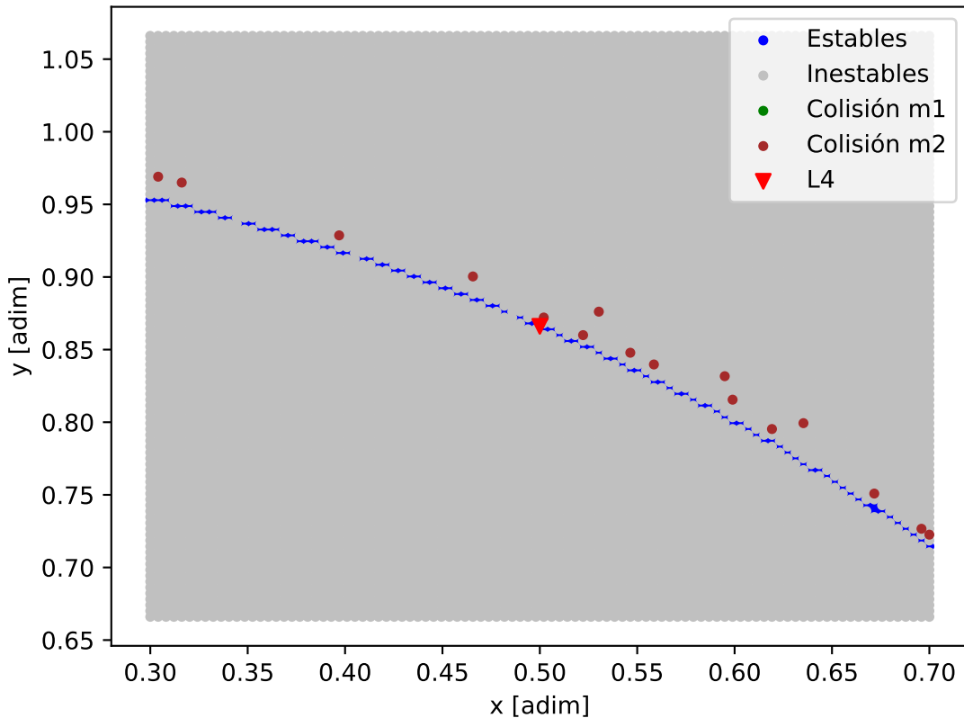
Mapa de estabilidad - Kepler-114_Kepler-114_c
