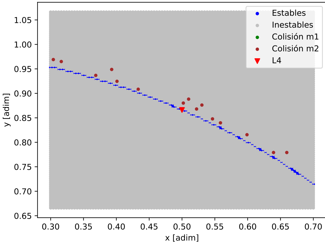
Mapa de estabilidad - Kepler-114_Kepler-114_d
