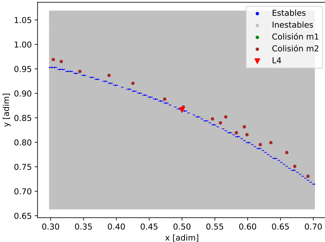
Mapa de estabilidad - Kepler-138_Kepler-138_c
