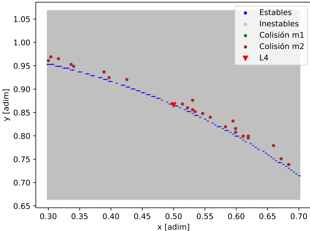
Mapa de estabilidad - Kepler-138_Kepler-138_d
