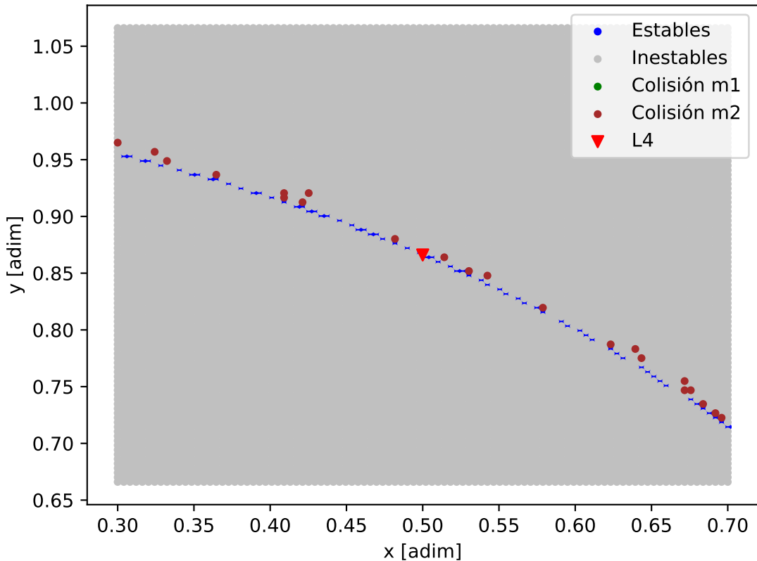
Mapa de estabilidad - Kepler-138_Kepler-138_e
