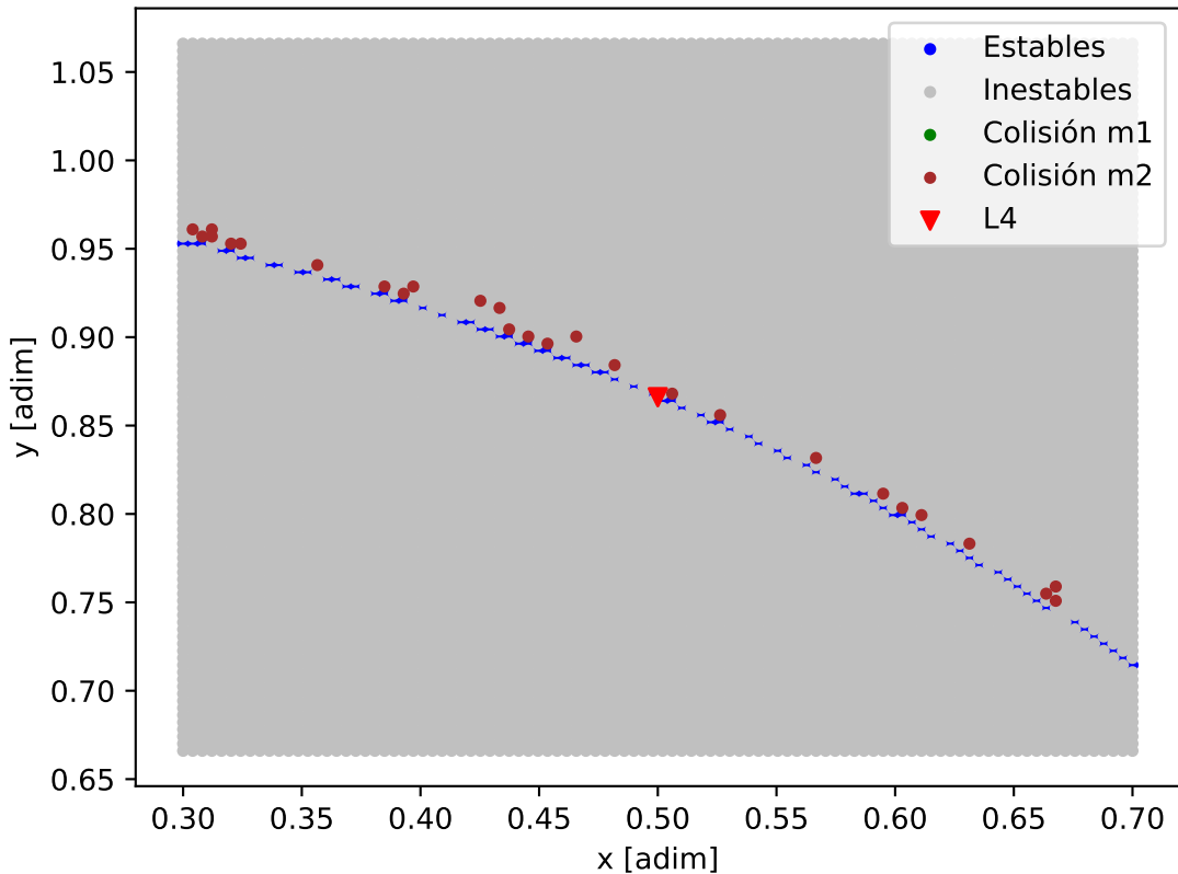
Mapa de estabilidad - Kepler-186_Kepler-186_b
