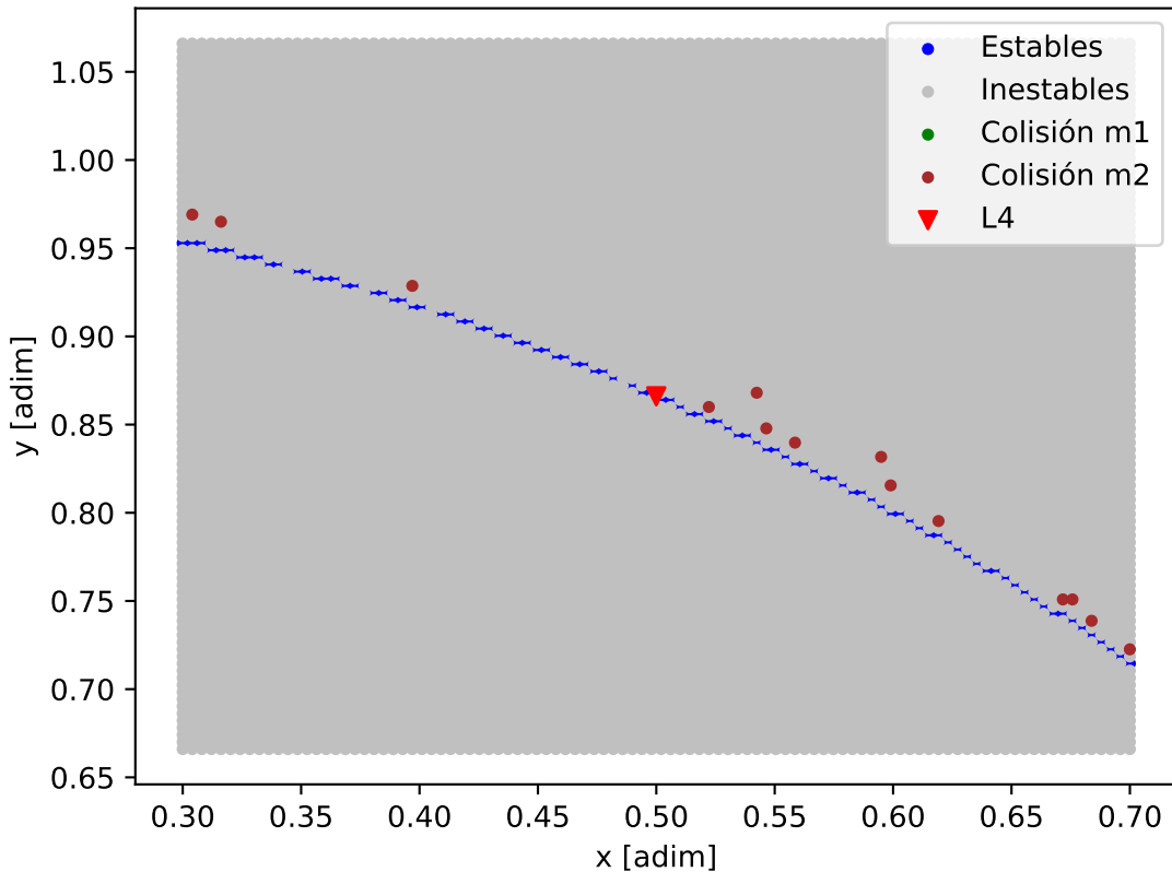
Mapa de estabilidad - Kepler-186_Kepler-186_d
