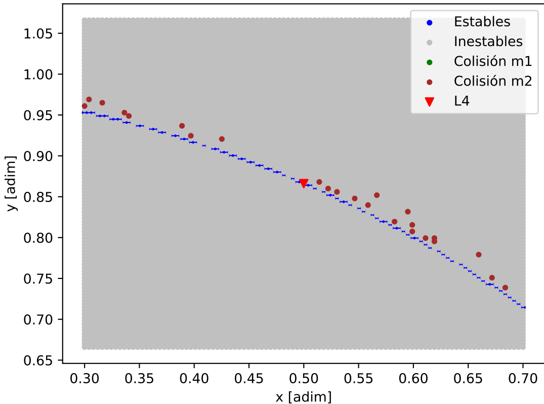
Mapa de estabilidad - Kepler-186_Kepler-186_e
