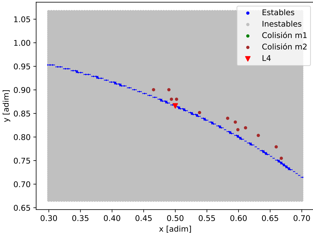
Mapa de estabilidad - Kepler-235_Kepler-235_b
