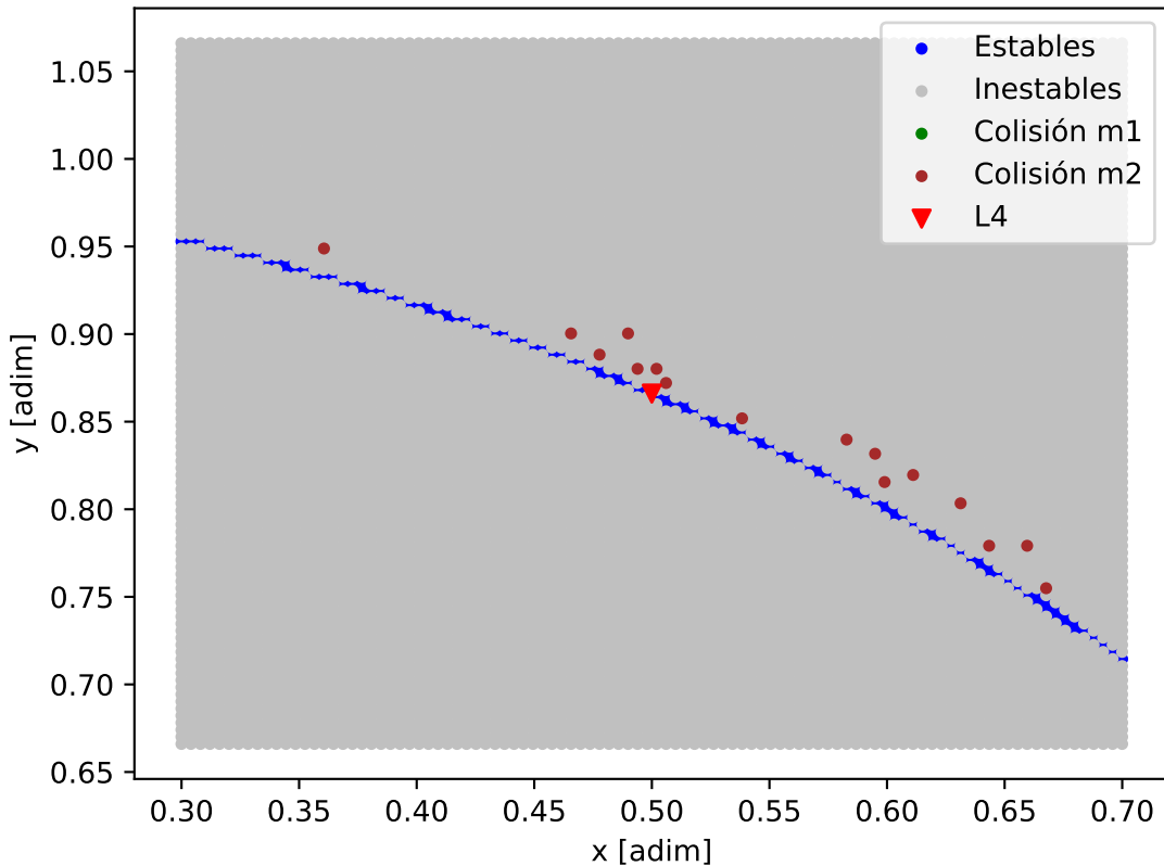
Mapa de estabilidad - Kepler-235_Kepler-235_e
