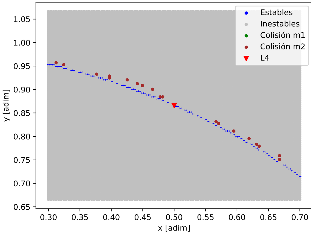
Mapa de estabilidad - Kepler-249_Kepler-249_b
