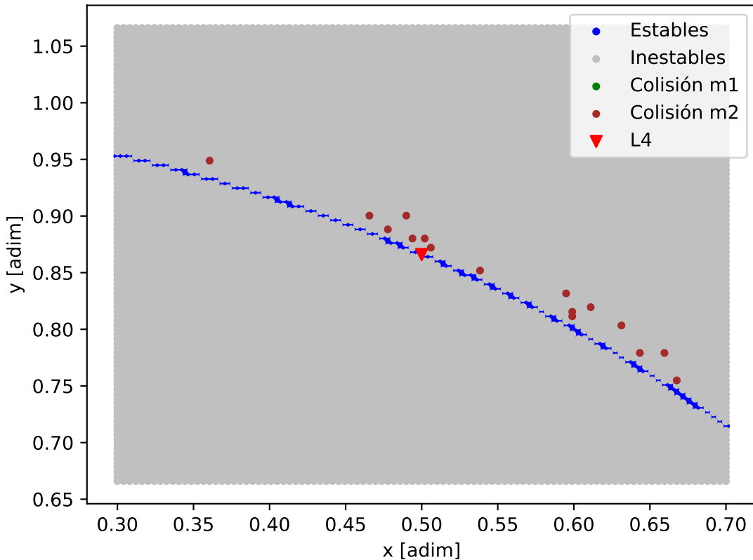
Mapa de estabilidad - Kepler-26_Kepler-26_b
