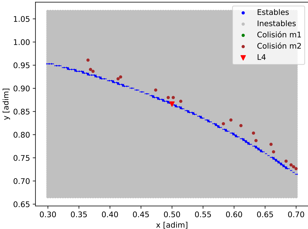
Mapa de estabilidad - Kepler-26_Kepler-26_c
