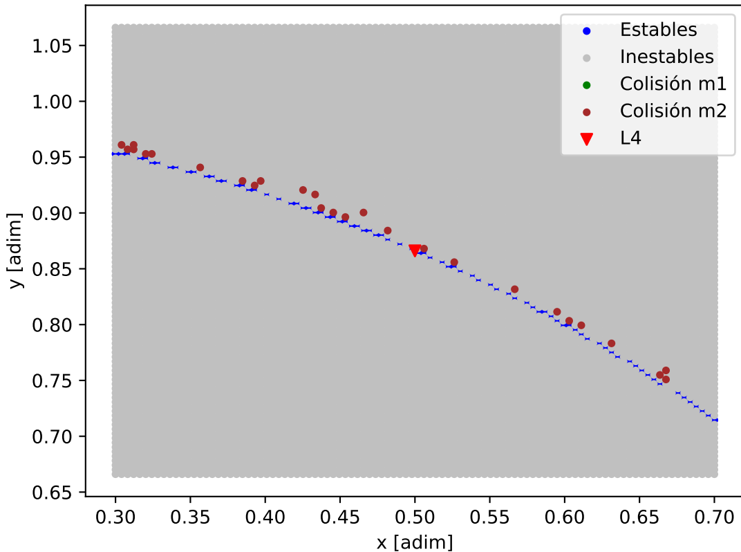
Mapa de estabilidad - Kepler-26_Kepler-26_d
