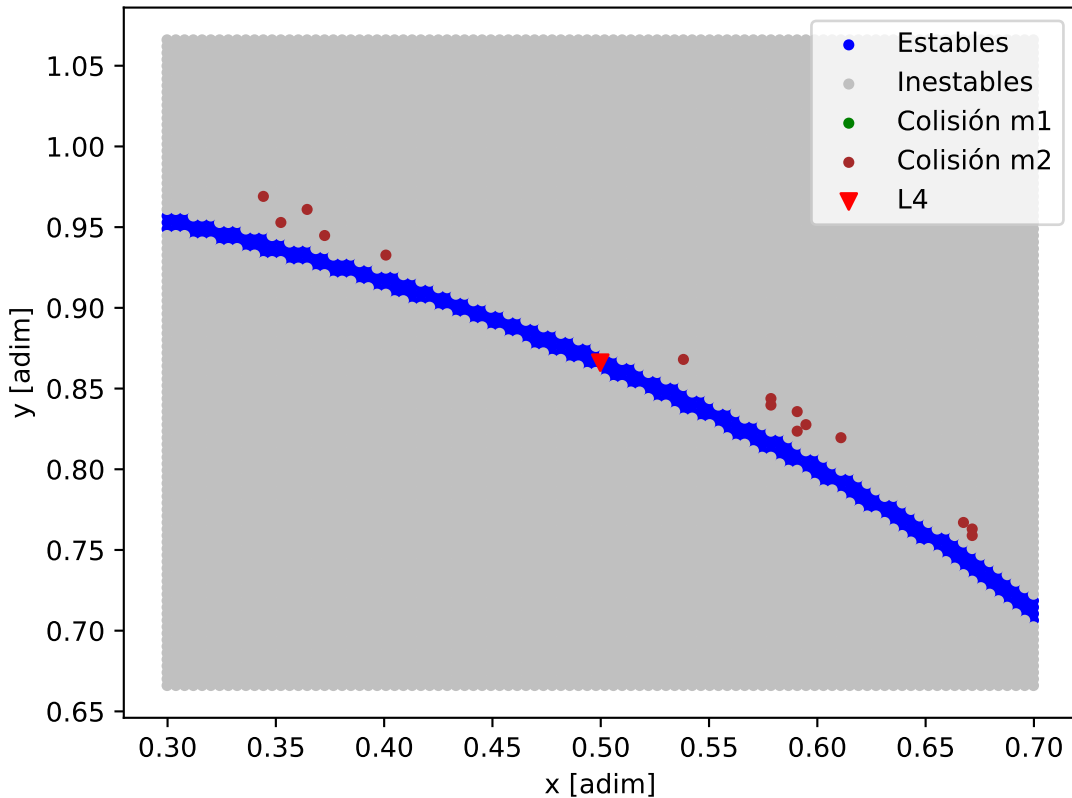
Mapa de estabilidad - Kepler-267_Kepler-267_b
