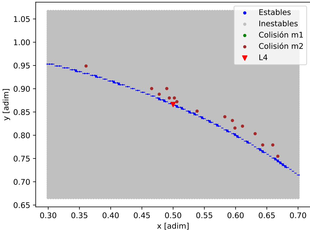
Mapa de estabilidad - Kepler-267_Kepler-267_c
