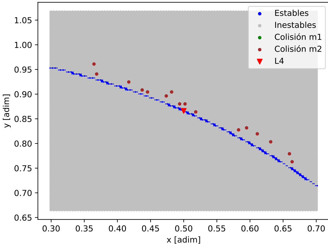
Mapa de estabilidad - Kepler-267_Kepler-267_d
