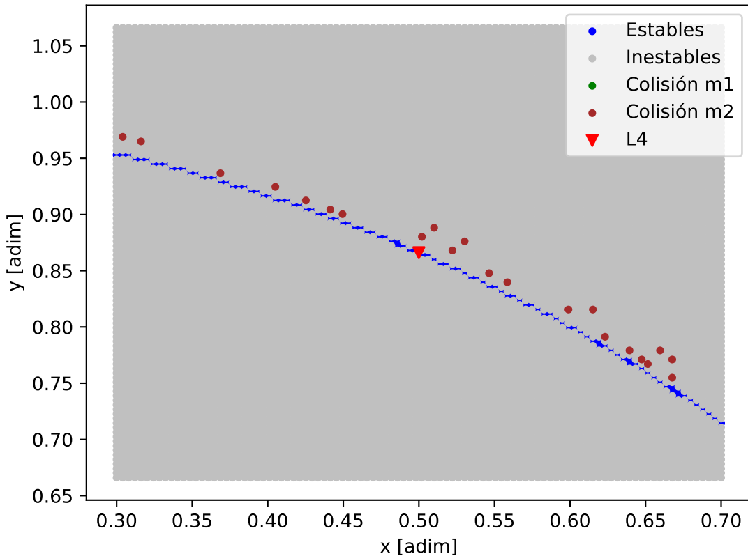
Mapa de estabilidad - Kepler-296_Kepler-296_b
