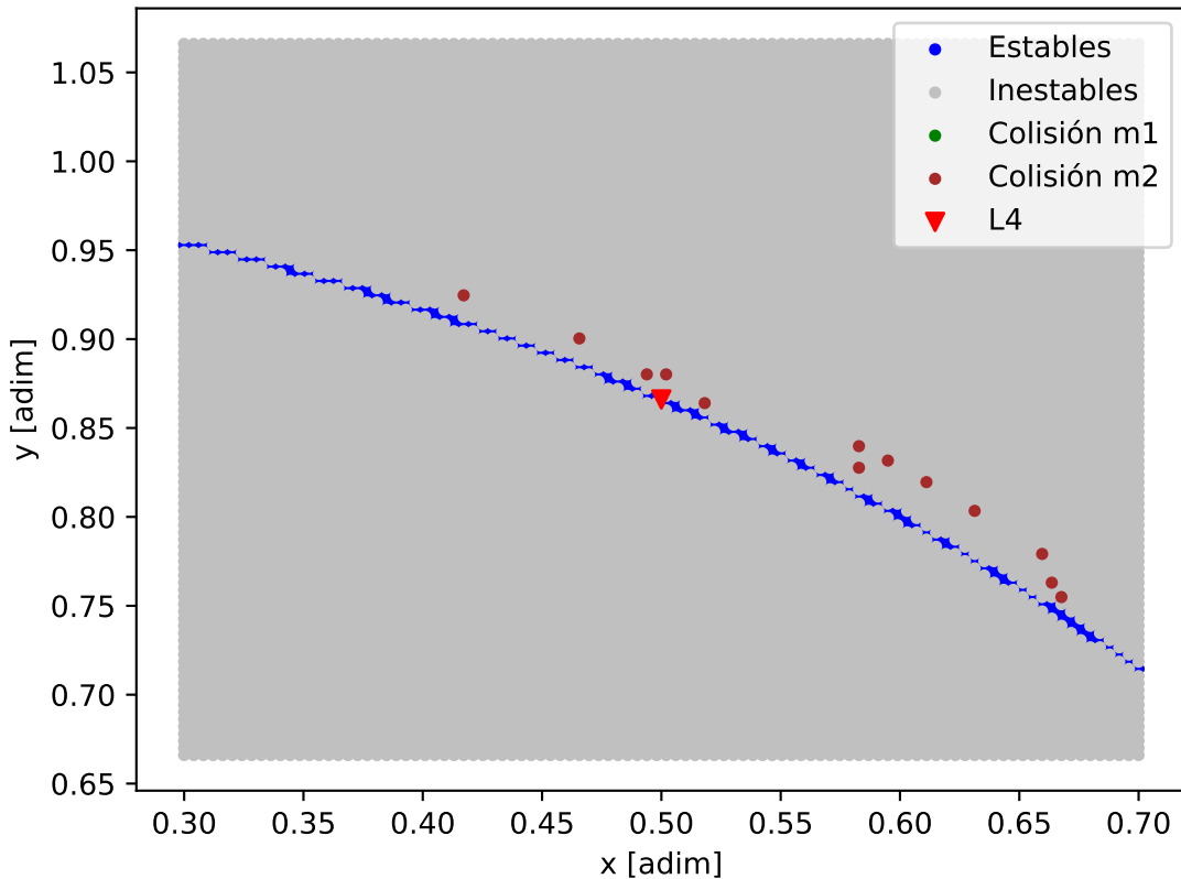
Mapa de estabilidad - Kepler-296_Kepler-296_d
