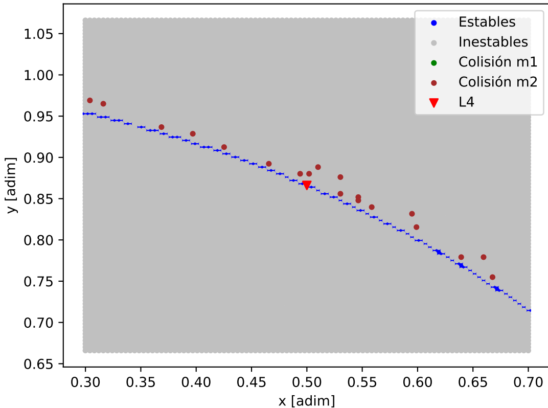
Mapa de estabilidad - Kepler-296_Kepler-296_e
