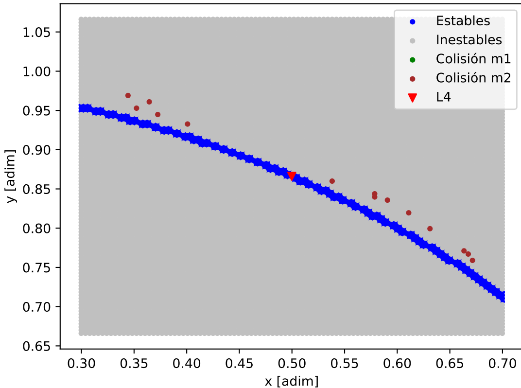
Mapa de estabilidad - Kepler-32_Kepler-32_d
